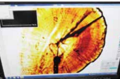
パソコン画面、木の年輪のように見えるのが、「鮎の耳石」です。
